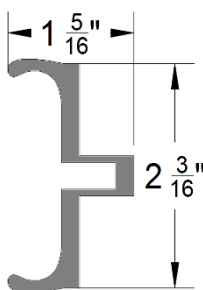
Edge Mount Handle Manija montada al borde
