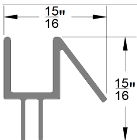
Drip Cap Tapa de goteo
