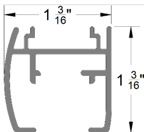
Header/Base Cabecero/Base
